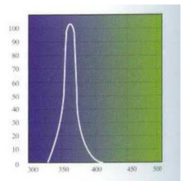
Emissionsspektrum der blauen UV Schwarzlicht-Röhre
